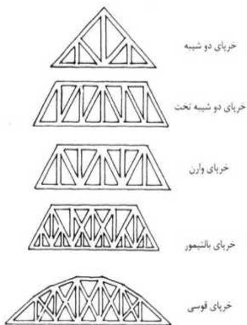
شکل ۳-۲۷ خرپاها
