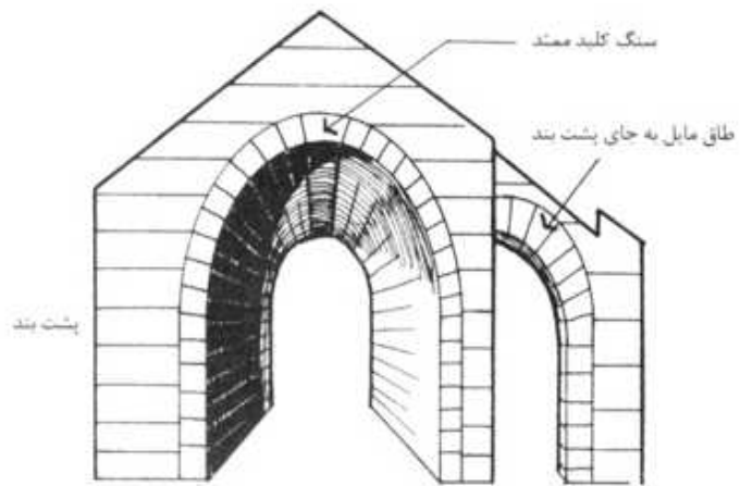
شکل ۲۲-۳ طاق چلیک
