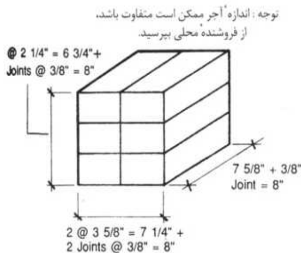
شکل ۳-۳ یک مدولار
