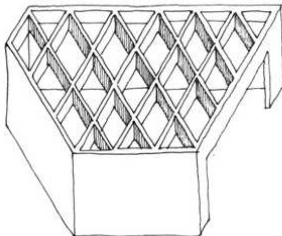
شکل ۳-۱۶ شبکه مایل
