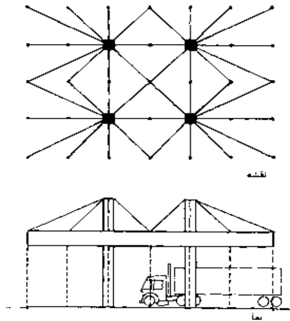
شکل ۳-۳۱ سازه‌های کابلی
